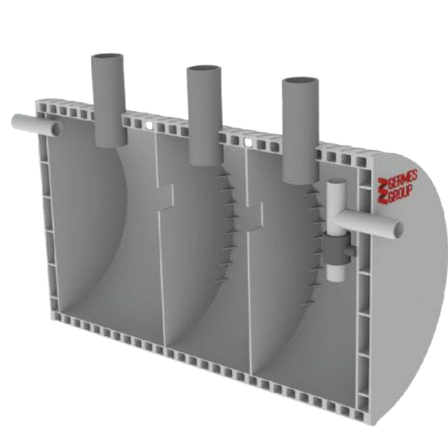
化粪池
