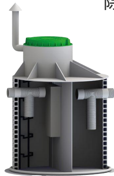
油脂分离器
